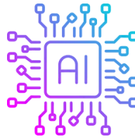
AI General
